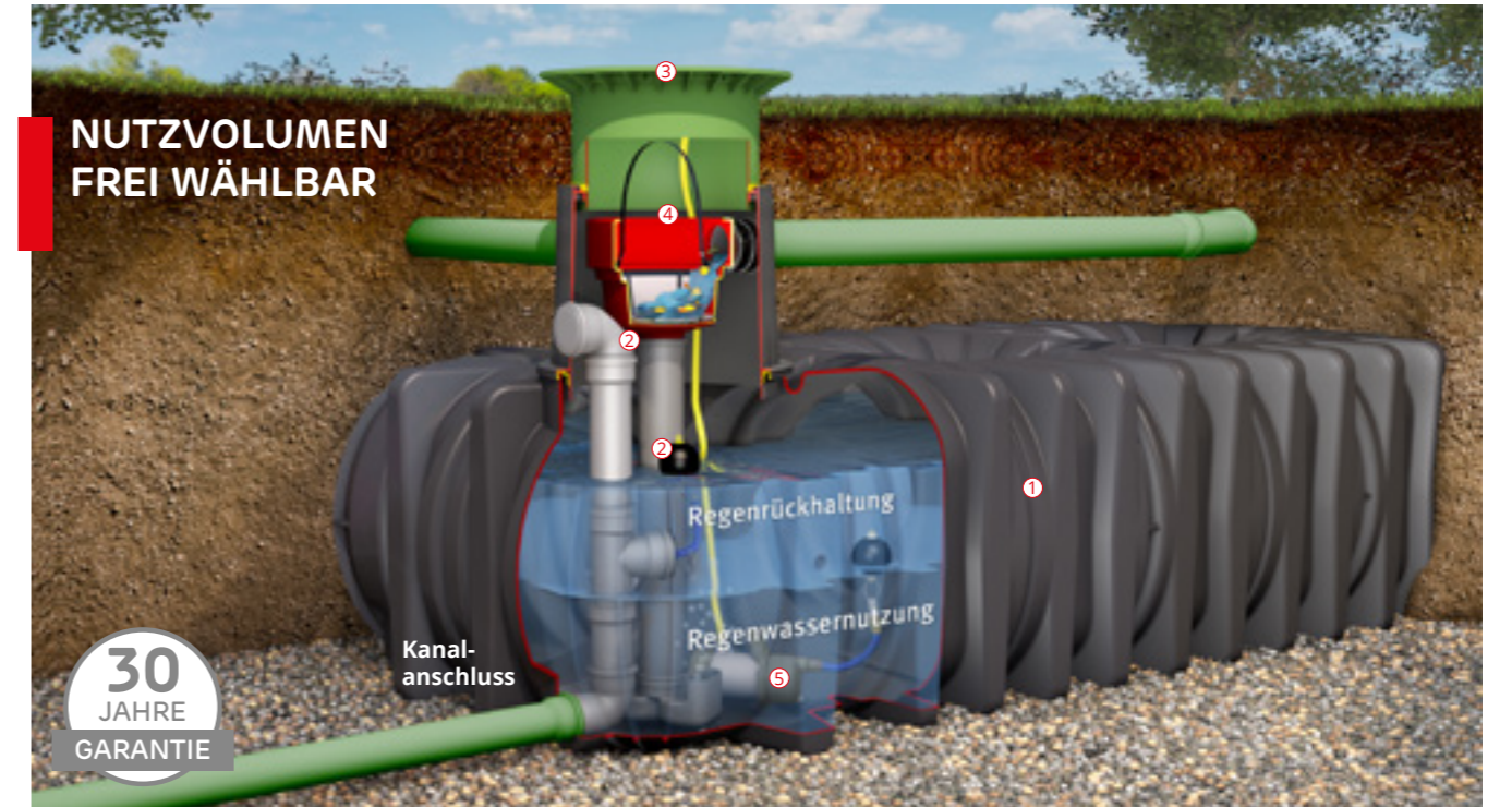
Abb. zeigt Platin XL Retentionszisterne mit Platin XL/XXL Retention Ausbaupaket 2 (Zubehör unten) und Technikpaket Garten-Komfort (Zubehör Seite 42)
