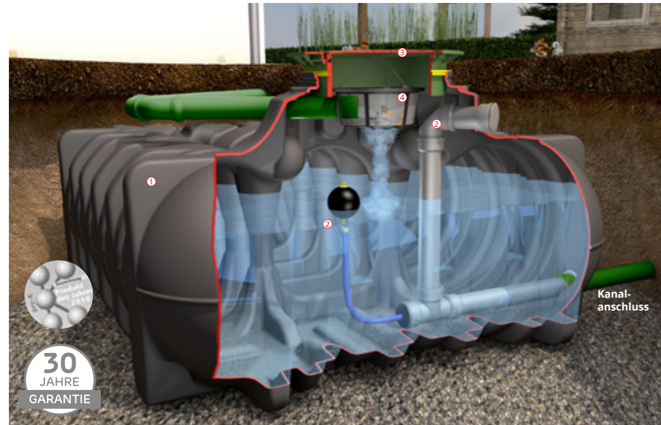
Abb. zeigt Platin Retentionszisterne mit Platin Retention Ausbaupaket 2 (Zubehör unten)
