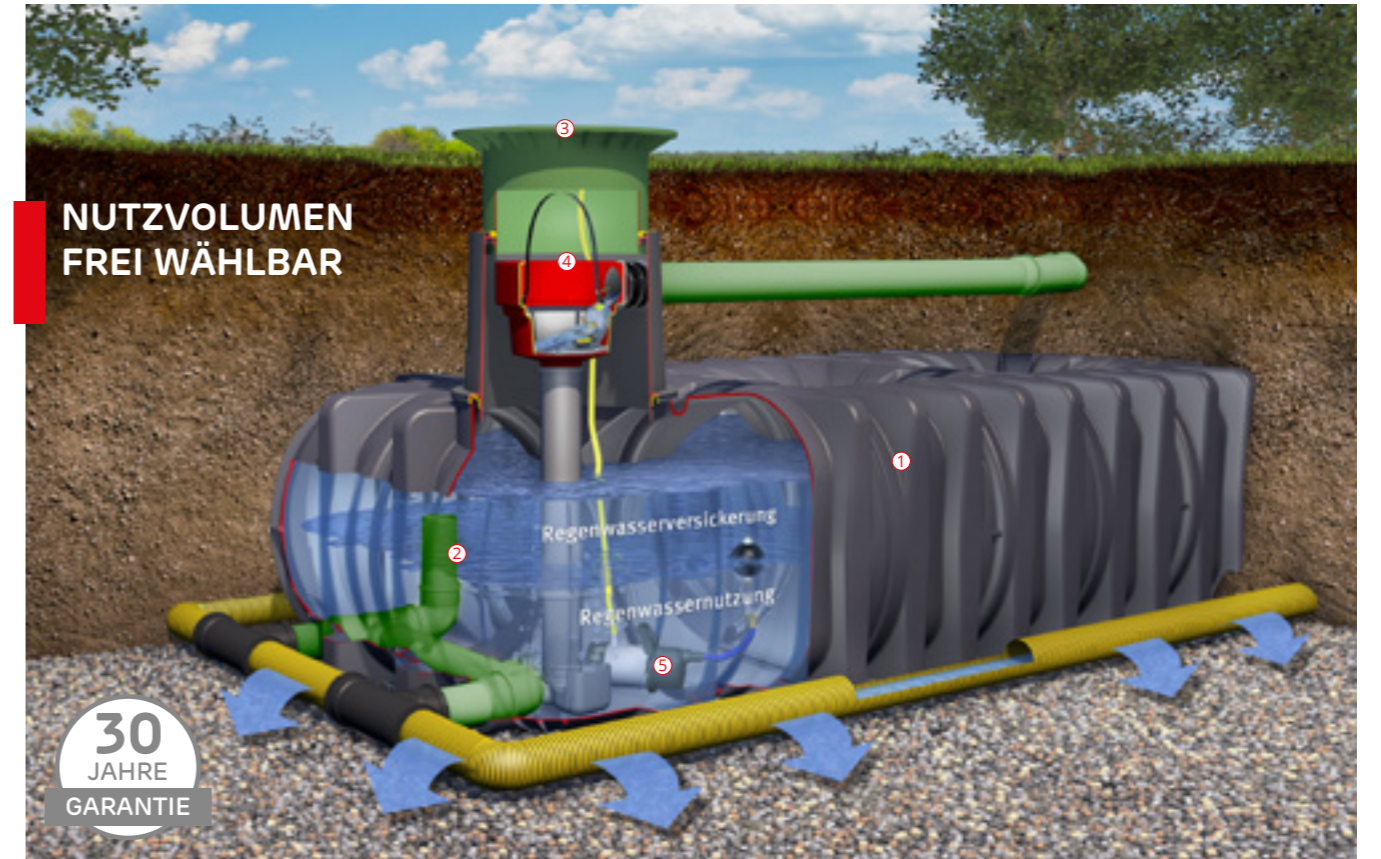
Abb. zeigt Platin XL Versickerung Plus mit Platin XL Retention/Versickerung Ausbaupaket 2 (siehe Zubehör) und Technikpaket Garten-Komfort (Seite 42)
