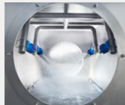
Funktion Filter-Reinigungseinheit
