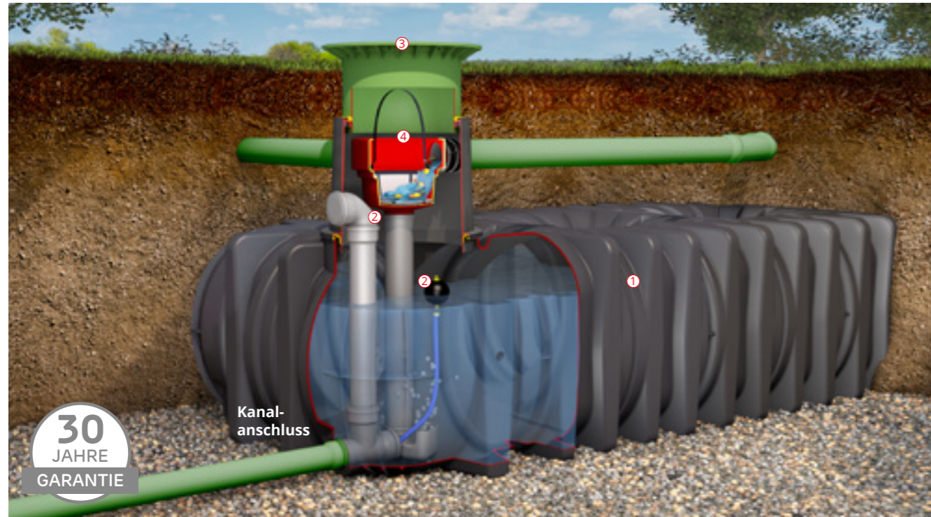
Abb. zeigt Platin XL Retentionszisterne mit Platin XL/XXL Retention Ausbaupaket 2 (Zubehör unten)
