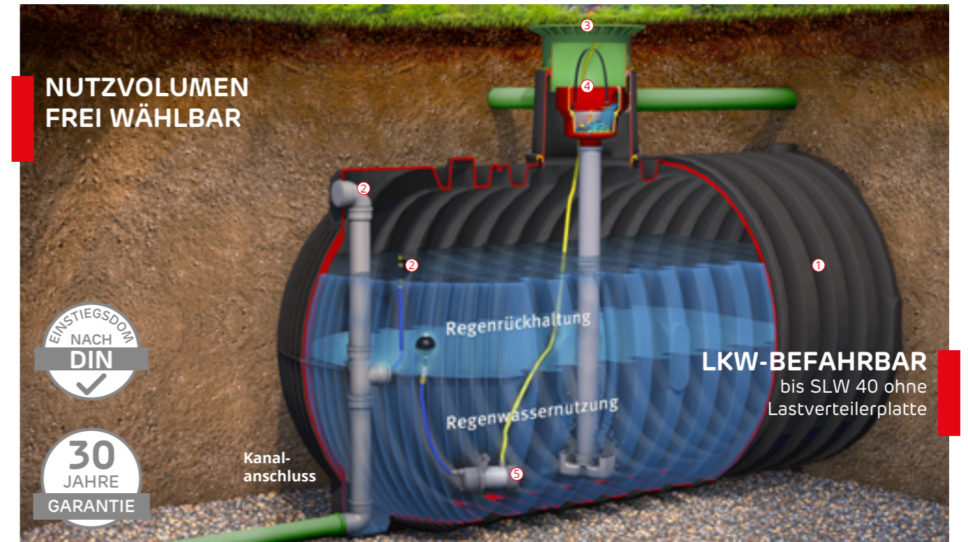
Abb. zeigt Carat XXL Retentionszisterne Plus mit Carat XL/XXL Retention Ausbaupaket 2 (Zubehör Seite 73) und Technikpaket Garten-Komfort (Zubehör S. 68)
