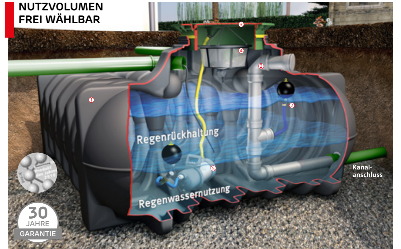
Abb. zeigt Platin Retentionszisterne Plus mit Platin Retention Ausbaupaket 2 (Zubehör unten) und Technikpaket Garten-Komfort (Zubehör Seite 42)
