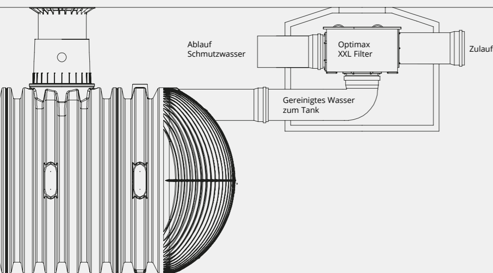
Funktion Filter-Reinigungseinheit
