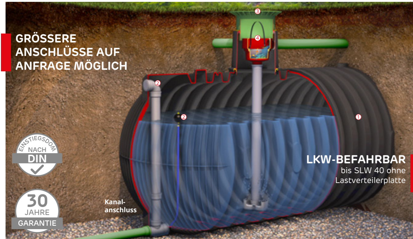
Abb. zeigt Carat XXL Retentionszisterne mit Carat XL/XXL Retention Ausbaupaket 2 (Zubehör Seite 77)
