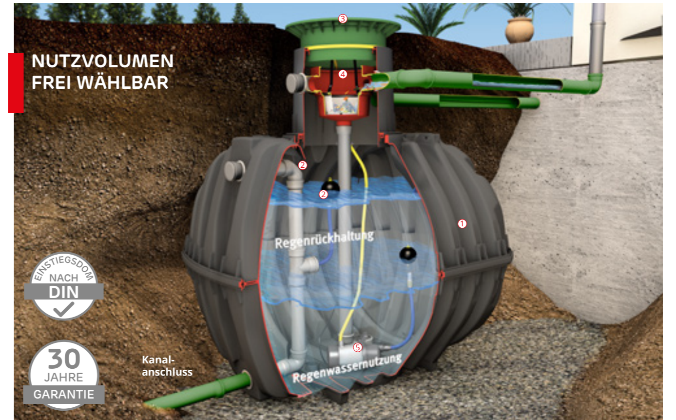
Abb. zeigt Carat Retentionszisterne Plus mit Carat Retention Ausbaupaket 2 (Zubehör unten) und Technikpaket Garten-Komfort (Zubehör Seite 68)
