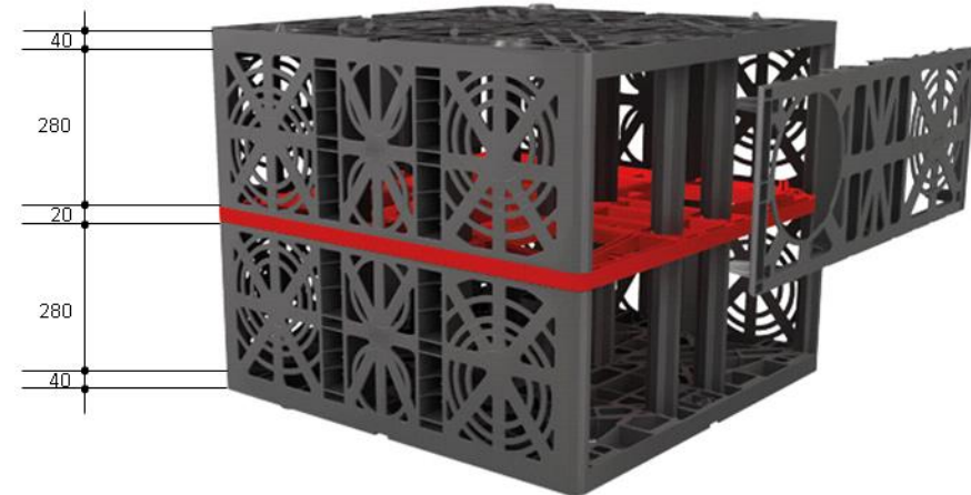
Drosselschacht
